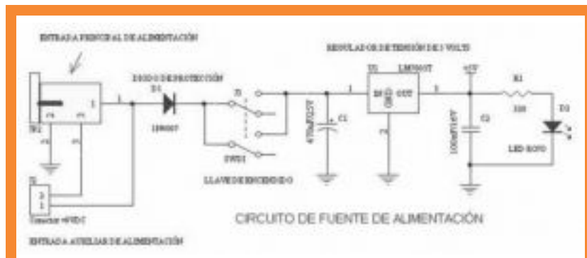
Esquemático de la fuente
