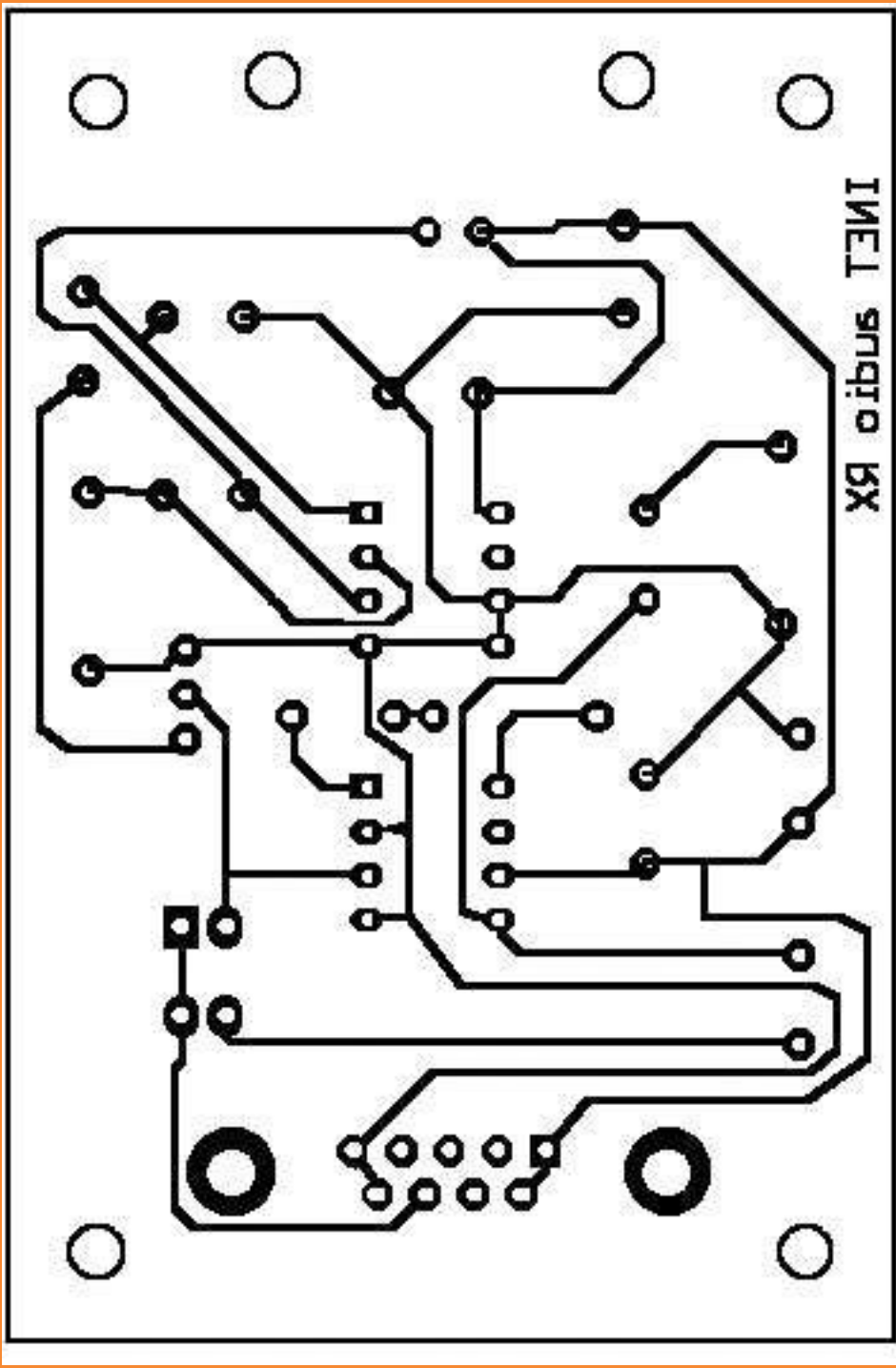
Placa receptora; lado sol- dadura
