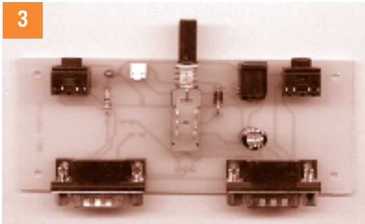
3 Montaje de diodo de protección contra inversión de polaridad, diodo LED, resistencia del diodo LED, capacitor de filtrado de fuente y conector auxiliar de alimentación
