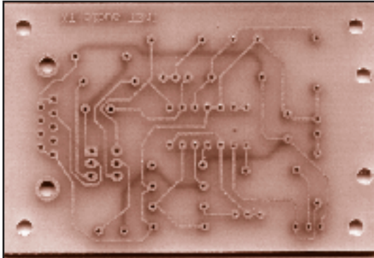
Placa del lado soldadura
