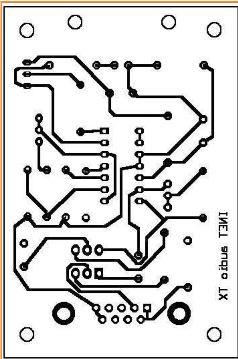
Placa transmisora; lado soldadura
