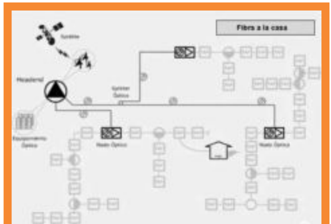
Esquema inicial de una red de CATV empleando fibra óptica
