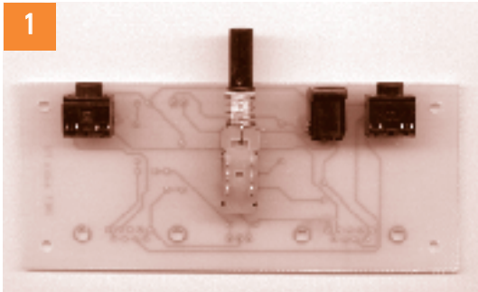
1 Montaje de llave de encendido, conectores de audio y conector de alimentación
