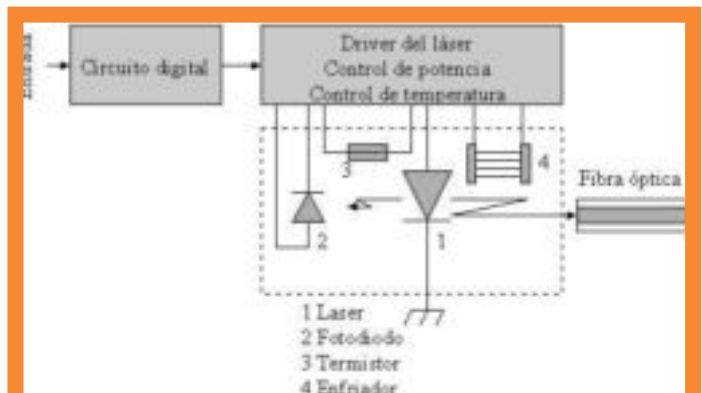
Diagrama en bloques de un transmisor analógico generalizado, basado en un láser
