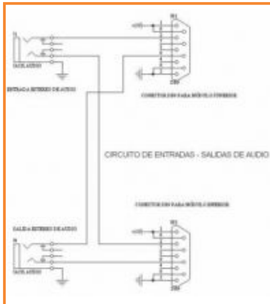
Esquemático del circuito
