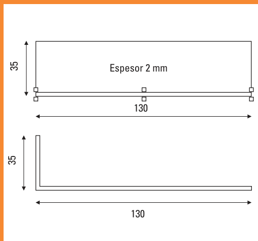
Vistas lateral y de frente de la base
