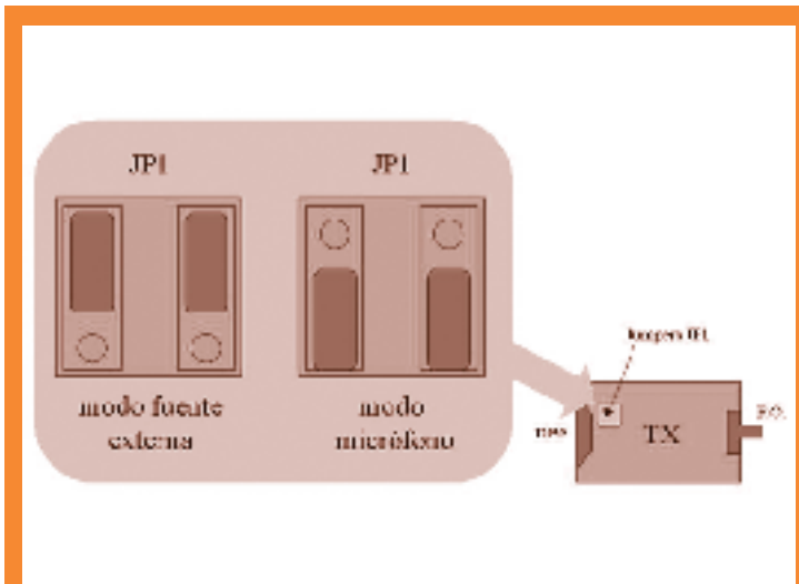
Posiciones que corresponden a cada modo de conexión
