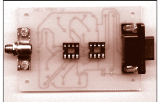
Montaje de conjunto conector RCA y chapa del interruptor Bisal, zócalo de integrados de 8 pines y conector DB9
