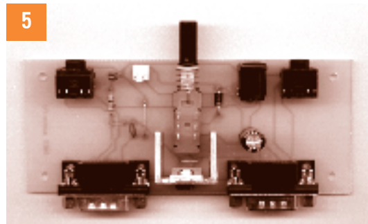
5 Montaje de regulador de tensión y dissipador de potencia; placa terminada
