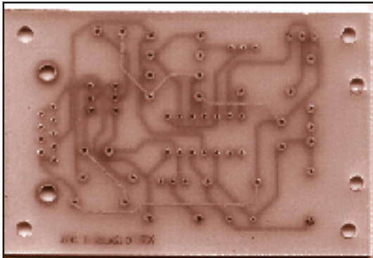
Placa del lado componentes
