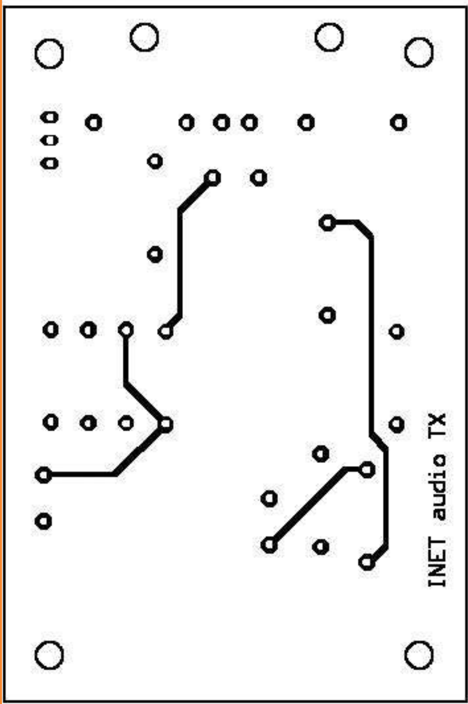
Placa transmisora; lado componentes
