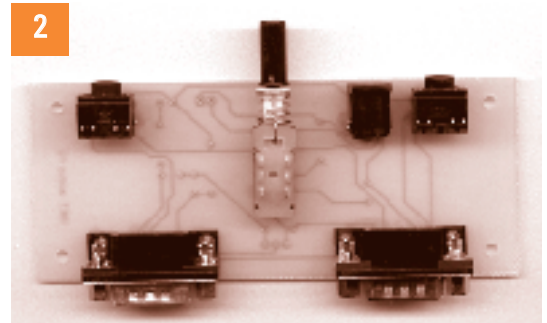
2 Montaje de conectores DB9 para interconexión con los módulos ópticos
