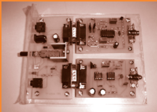
Detalle de la conexión de los módulos a cada placa principal
