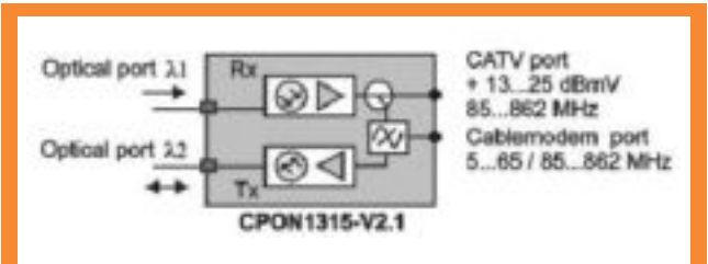
Circuito empleado en la recepción de la señal óptica que se transmite desde la cabecera de la red de CATV
