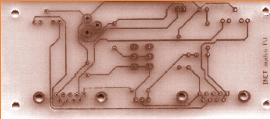
Circuito impreso del lado soldadura o cobre
