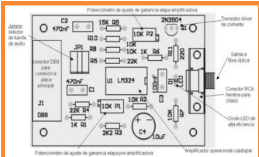
Esquema de la placa del transmisor óptico digital
