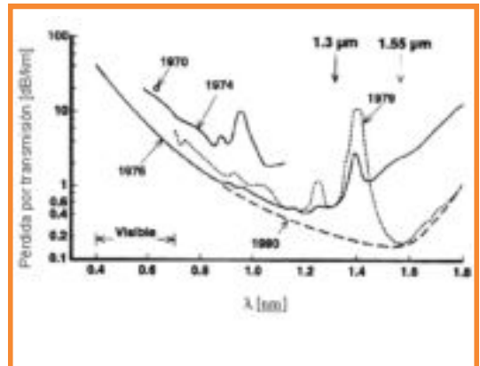
Evolución de las pérdidas de potencia luminosa por unidad de longitud
