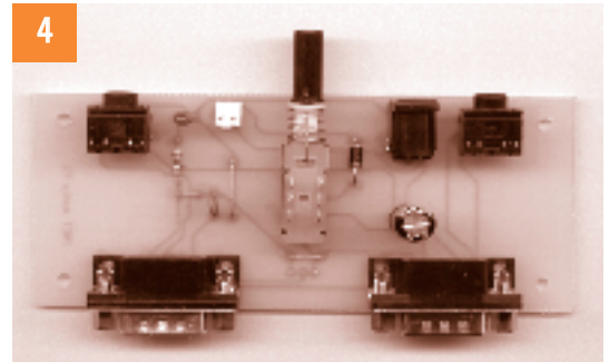
4 Montaje de capacitor de salida del regulador y puentes; lado componentes
